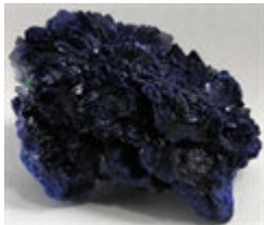
Azurite crystal cluster, Yang Chun Mine, Guangdong Province, China.
